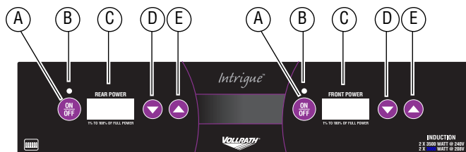
Panneau de commande du modèle sur comptoir 59522, 6954702, 6954703, 6954704
