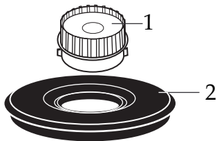
500664 2 Piece Lid
