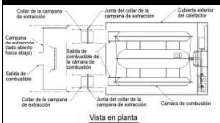
Figura 10 - Instalación de la campana de extracción
