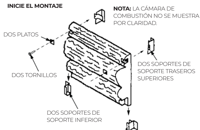
FIGURA 21 - INICIE EL MONTAJE
