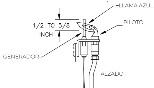
FIGURA 18- CARACTERÍSTICAS DE LA LLAMA DEL QUEMADOR
