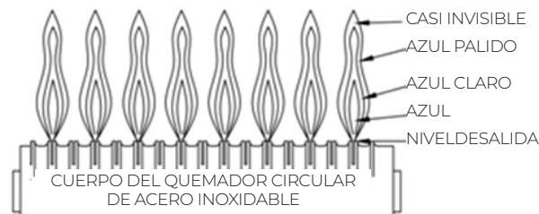
FIGURA 18- CARACTERÍSTICAS DE LA LLAMA DEL QUEMADOR
