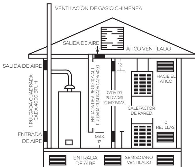
FIGURA 10 - AIRE DEL EXTERIOR O SEMISÓTANO
