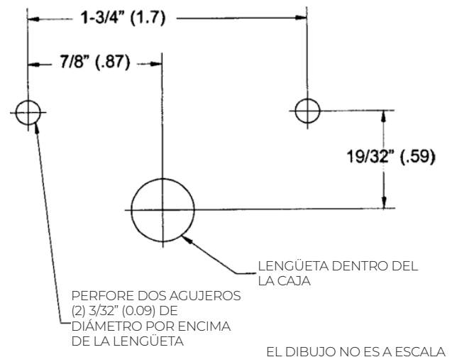
FIGURA 13 - AGUJEROS DE TERMINACIÓN
