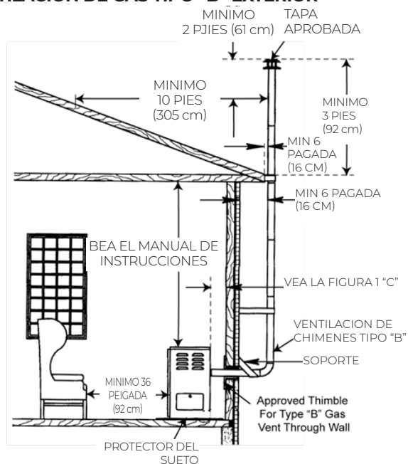
FIGURA 16 B - VENTILACIÓN ALTERNA
