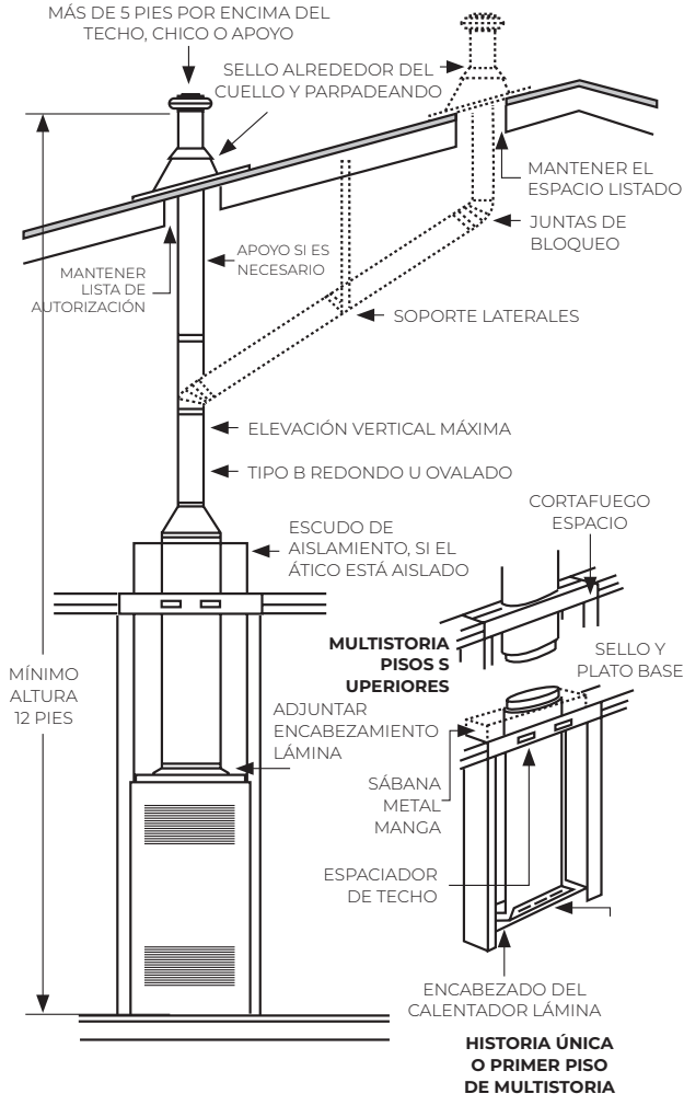
FIGURA 16 B - VENTILACIÓN ALTERNA
