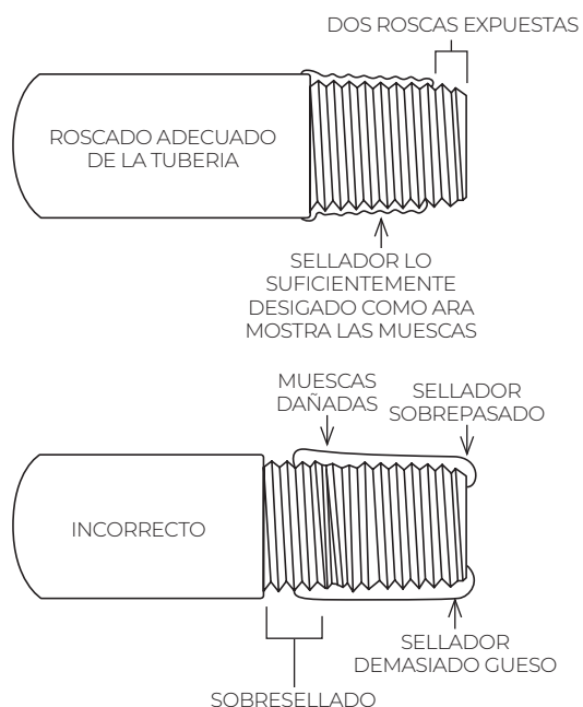
FIGURE 3 – PRÁCTICA DE CANALIZACIÓN ADECUADAS
