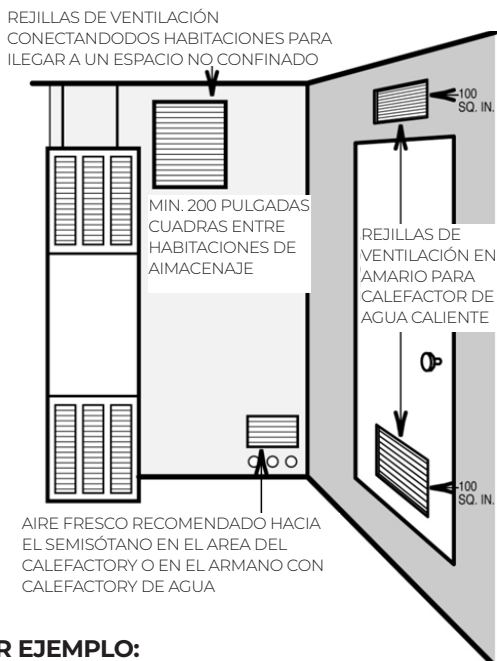
FIGURA 9 - REJILLAS CONECTANDO HABITACIONES PARA FORMAR UN ESPACIO NO
