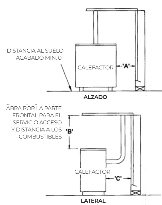
FIGURA 1 - DISTANCIAS MINIMAS REQUERIDAS
