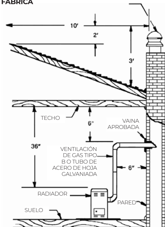
FIGURA 14 - VENTILACIÓN A UNA CHIMENEA DE FABRICA
