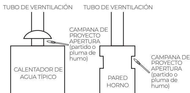
FIGURA 6 - DERRAME DEL EXTRACTOR
