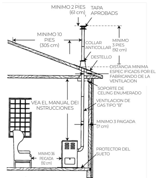
FIGURA 15 - PONGA RECTA LA VENTILACIÓN CON LA VENTILACIONE DE GAS TIPO "B"
