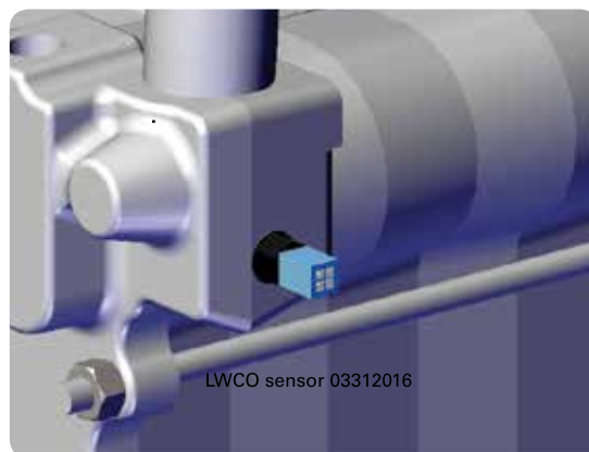
Illustration 9 Coupure de bas niveau d'eau de type intégré
