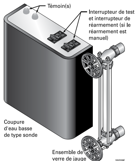
Illustration 8 Coupure d'eau basse de type sonde
