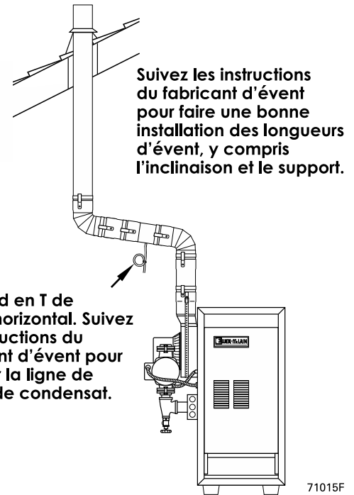
Illustration 13 Évacuation directe évacuation verticale
