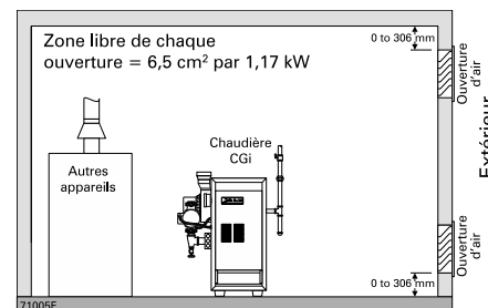
Illustration 3 Air qui provient directement de l'extérieur
