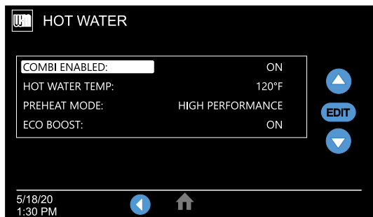
Figure 11 Affichage de la commande de la chaudière ECO Tec Commandes combinées du propriétaire
