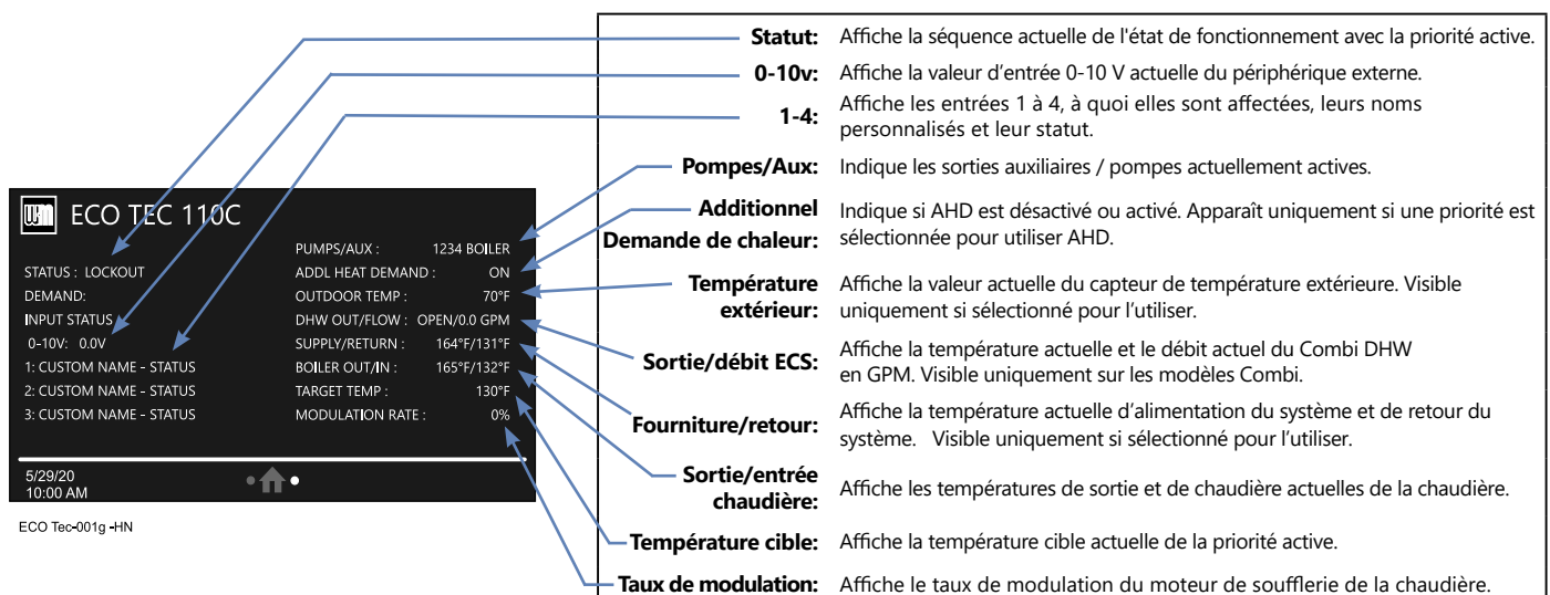
Figure 7 L'afficheur de commande de la chaudière ECO Tec indique
