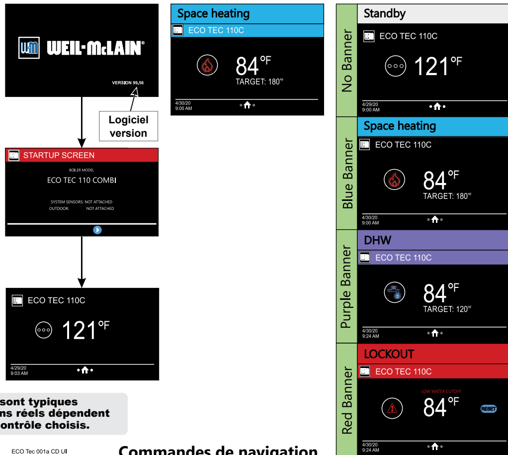
Figure 6 L'afficheur de commande de la chaudière ECO Tec indique
