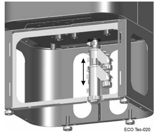
Figure 3 Piège à condensats de la chaudière (panneau d'accès avant retiré)
