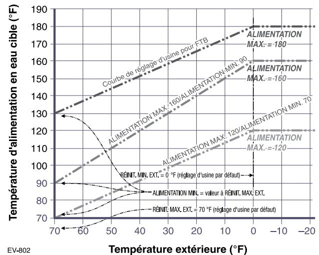
Figure 55 Fonctionnement de la réinitialisation extérieure
