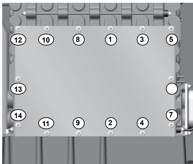
Figure 89 Séquence de serrage des écrous – SF-750 Serrer progressivement les écrous, en répétant la séquence indiquée ci-dessous jusqu'à atteindre un couple de 160 inch-pounds +/- 10 inch-pounds / 18 N-m +/- 1 N-m
