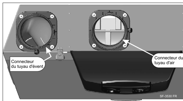
Figure 40 Raccordements d'air et d'évent de la chaudière
