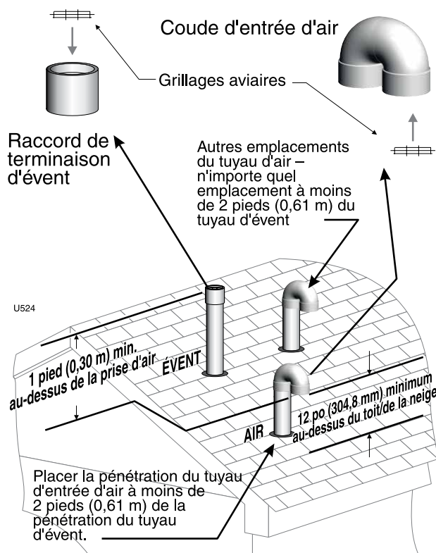
Figure 38 Terminaison verticale – Tuyaux séparés
