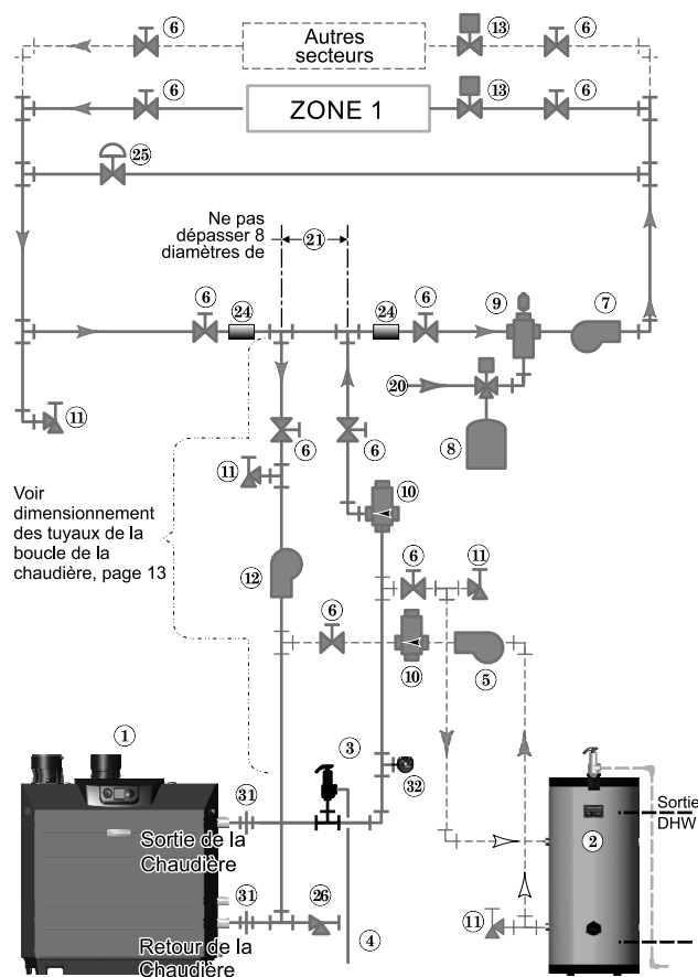
Figure 7 Zonage avec soupapes de secteur plus tuyauterie DHW en option
