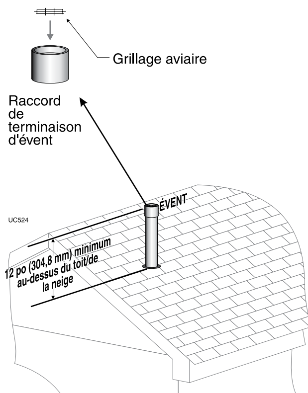
Figure 25 ÉVACUATION DIRECTE – Terminaison verticale
