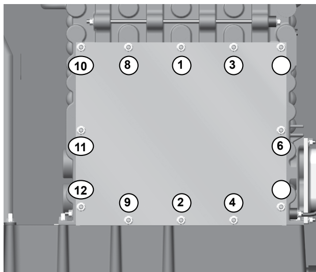
Figure 88 Séquence de serrage des écrous – SF-550 Serrer progressivement les écrous, en répétant la séquence indiquée ci-dessous jusqu'à atteindre un couple de 160 inch-pounds +/- 10 inch-pounds / 18 N-m +/- 1 N-m
