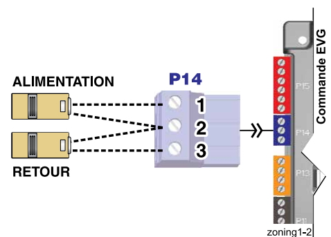
Fixer à la tuyauterie d'alimentation et de retour
