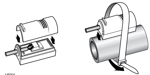
Fixer à la tuyauterie d'alimentation et de retour
