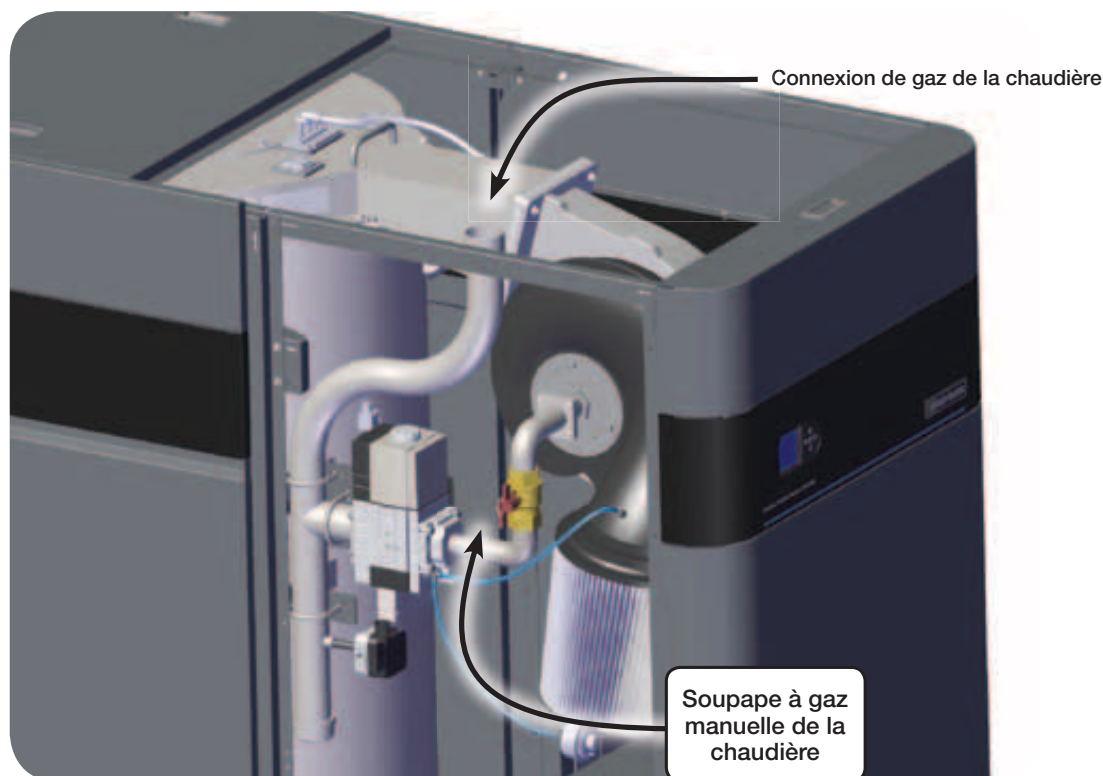
Figure 3 Emplacement de la soupape à gaz manuelle de la chaudière SVF-2000 , panneau supérieur retiré
